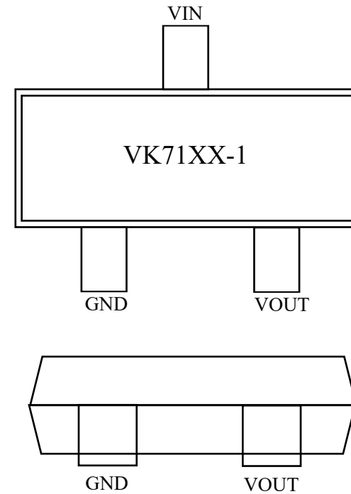
SOT23-3
