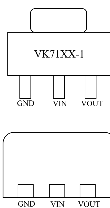
SOT-89
